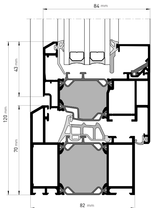
heroal W 72 CL, Schnittdarstellung
